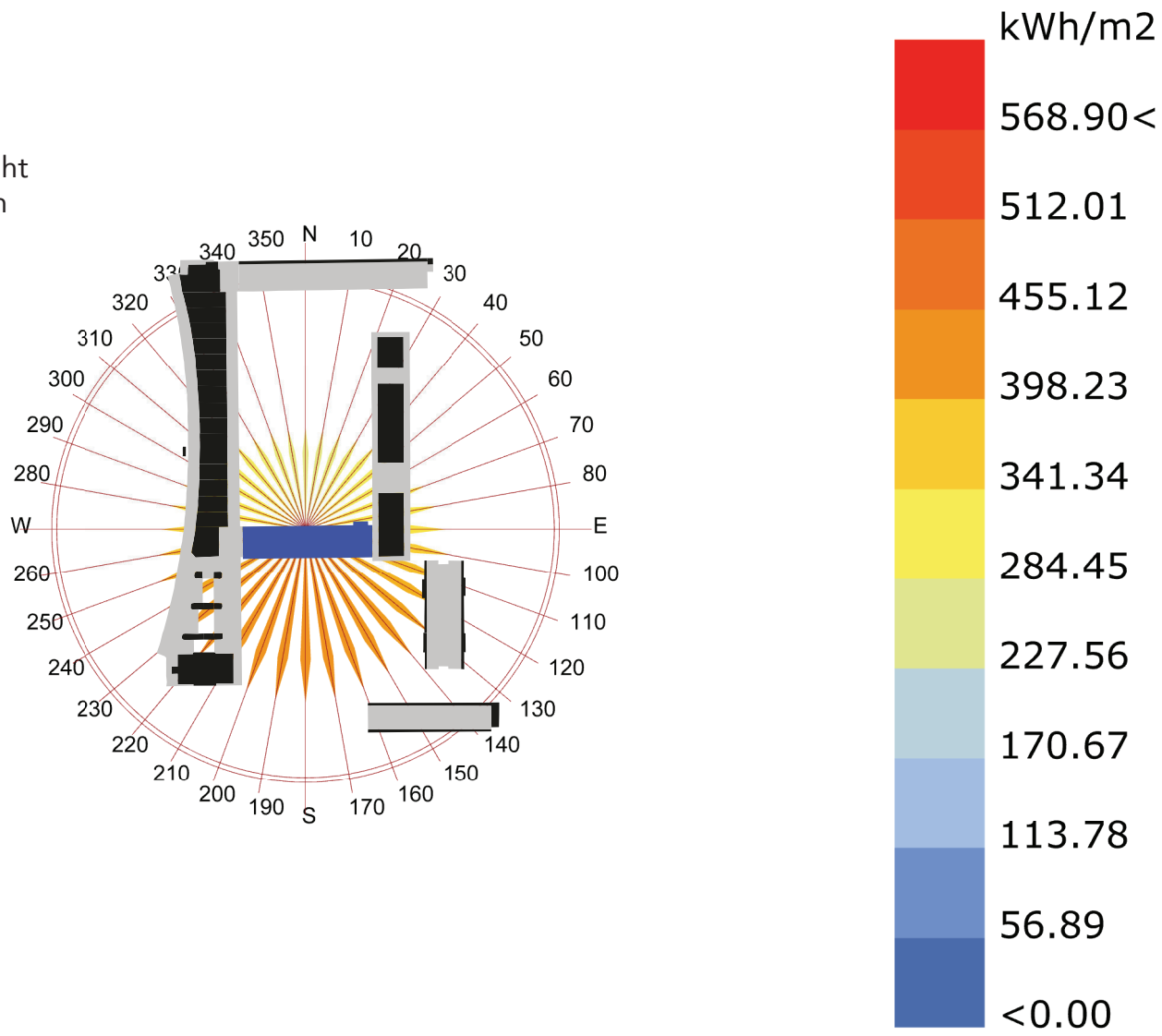
Diffuse Radiation(kWh/m2) London_ON_CAN_1975 1 JAN 1:00 - 31 DEC 24:00
